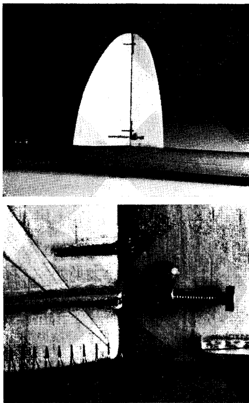
Bild 4 och 5. Sidorodrets utformning och detalj av gångjärn, stoppskruvar och fjäder ur 0,1 mm tråd.
