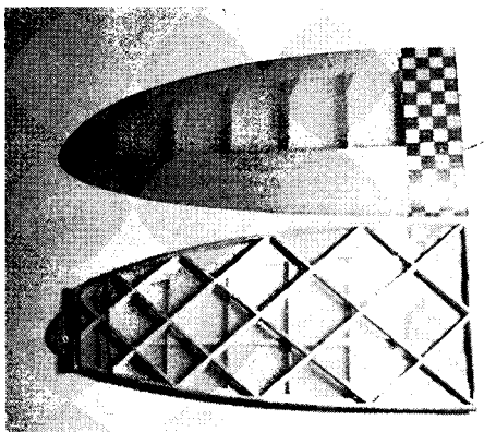
Bild 3. Spetsarna spännes fast med gummisnoddar på en vridstyv ram. Obs! att ena spetsen skall ligga plant, den andra (innerspetsen) skränktes med en liten klots under framkanten vid delningen.
