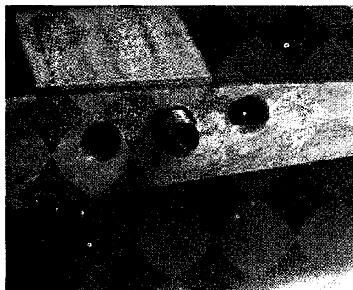
Bild 1 och 2. Sidovy och närbild av vingspetsen. Ett styrtstift på var sida om pianotråden som håller ihop spets och mittvinge. Styrtstift av kapad och filad skruv gängas direkt i plywoodsprygeln, och kan då lätt flyttas mellan de olika lägena.
