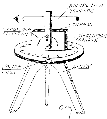
TEODOLIT - PRINCIPSSKISS
