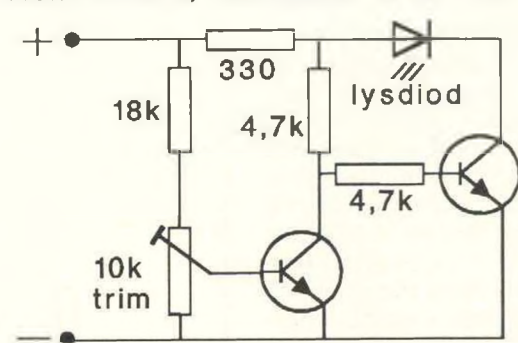
Transistor BC107, BC108 el likn Lysdiod av standardtyp
