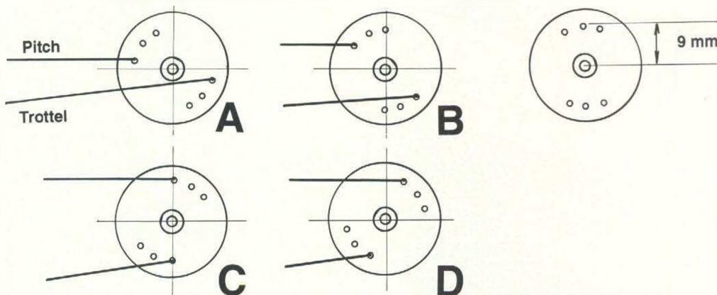
Skiss över kombinerat trottelt- & pitchservo. (Sitter på pitchservots ordinarie plats)
