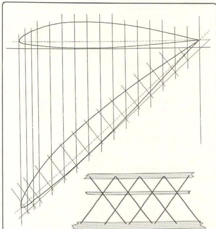
Skissen visar hur man överför en profil till geodetisk form.
