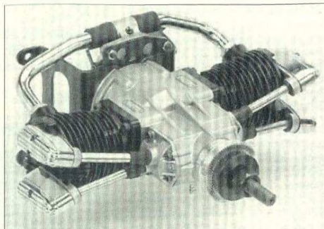
▲ FA 300 TL 50,0 cc • 1.660 g • 4,9 hk Pris 7.795:-
