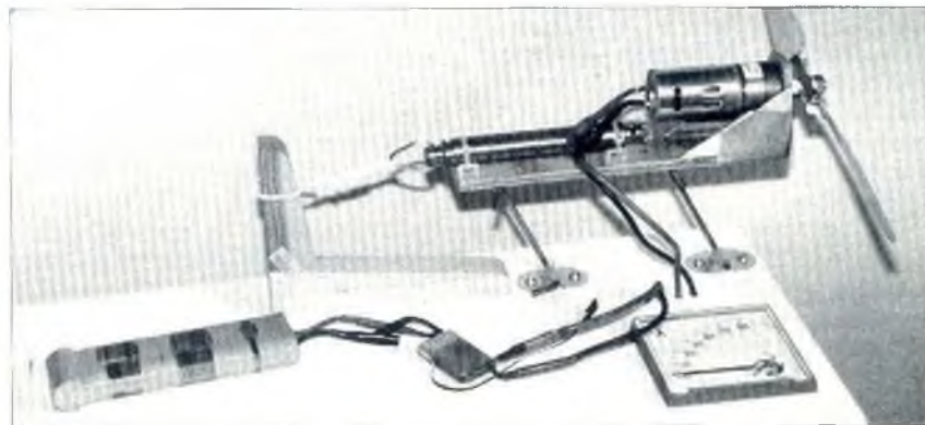
Rune Olssons mätanordning består av en enkel trävaggan där motorn sätts fast. På vaggan finns en dynamometer vars arm dras ut när vaggan dras åt höger av propellern. Strömmen mäts med en stor ampèremeter och strömmen regleras med ett vanligt fartreglage.
