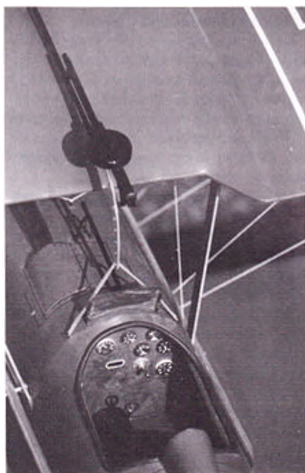
På billedet herunder ses maskingeværet fastgjort på øverste vinge, og på det lille billede til venstre ses, hvorledes fastlåsningsen af dette øverste maskingevær sker med gummibånd af hensyn til »slå-af-sikkerheden«.
