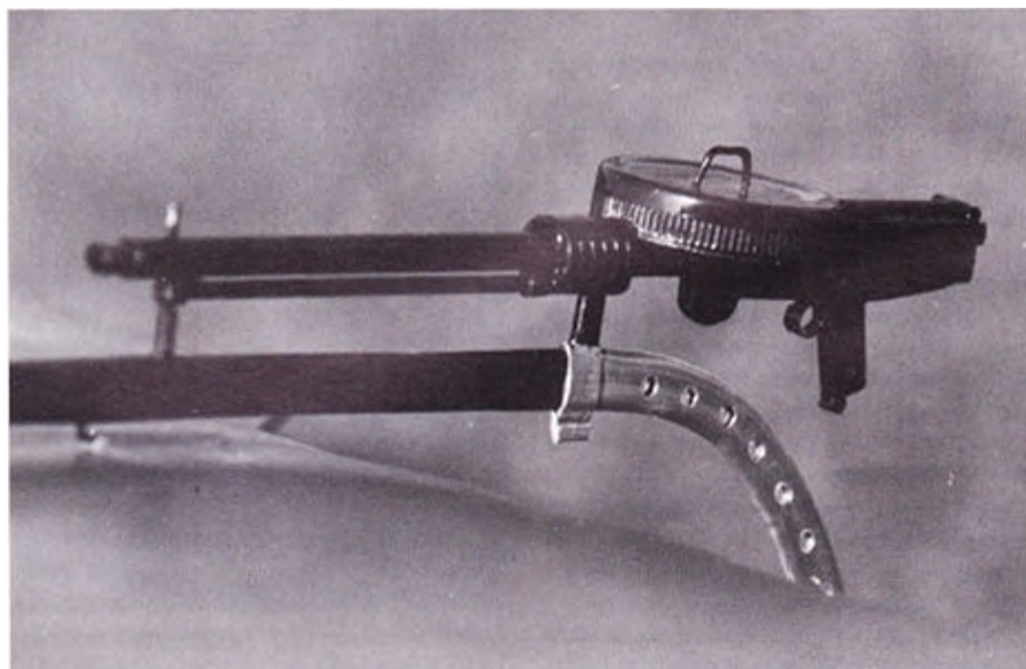
På billedet herunder ses maskingeværet fastgjort på øverste vinge, og på det lille billede til venstre ses, hvorledes fastlåsningsen af dette øverste maskingevær sker med gummibånd af hensyn til »slå-af-sikkerheden«.
