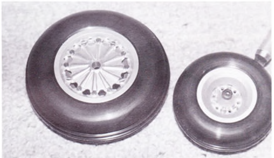
Håndlavede sælge med påmonterede dæk til bugstel og næsehjul.
