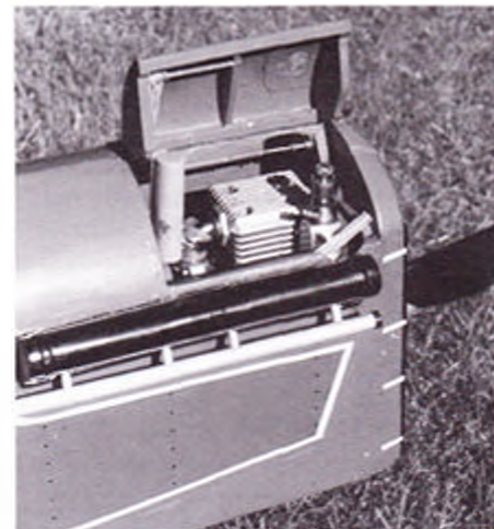
Motorrummet åbnes som på en veteranbil. Lukketøjet er almindelige gummibånd, og hele låget holdes på plads af en langsgående fjeder.
