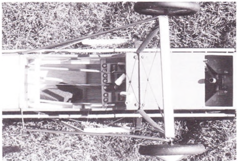
Hjulfastgørelse og køleluftafgang, hvor også udstødning og tanken erbort ud.
