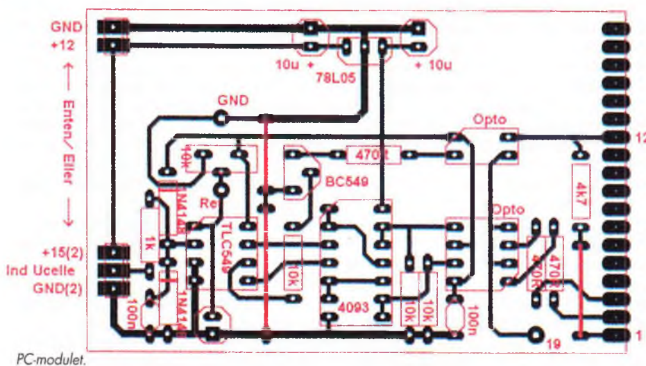
PC-modulet.
