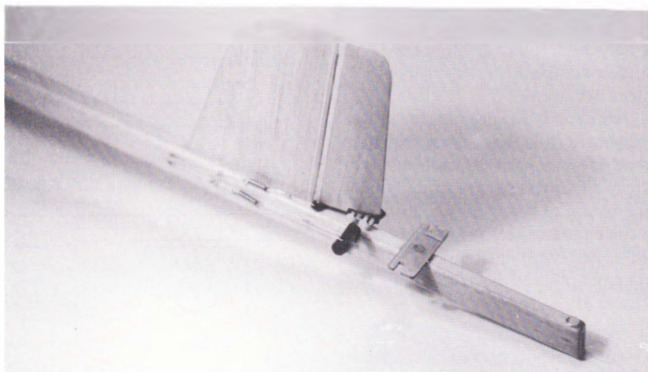
Vippearmen og skruerne på sideroret ses monteret på en »Blue Bird« A2-model. Delene ved halefinnen er alle af plastik og vejer knap 2 gram. I sættet medfølger også en trimskrue til haleplanet.
