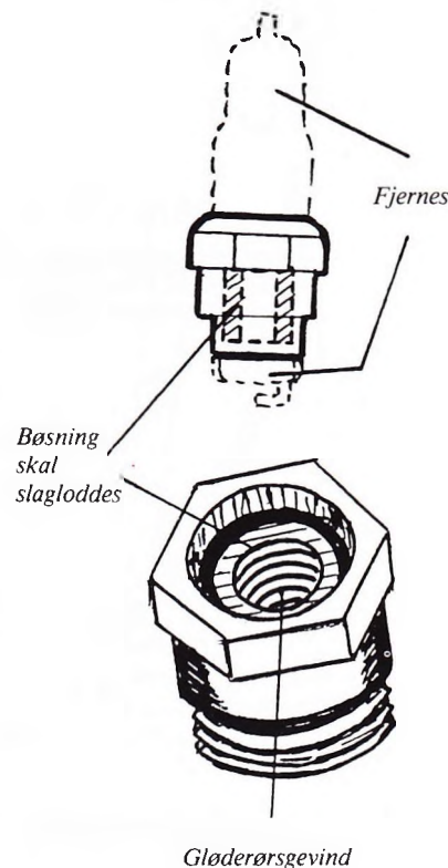
Fig. 2. Tændrør kan laves om til gløderør.
