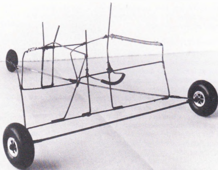
Startvognen på øverste billede er lavet sådan, at modellen ligger løst på den. Den nederste startvogn holder modellen fast og falder af, når modellen er kommet i luften.
