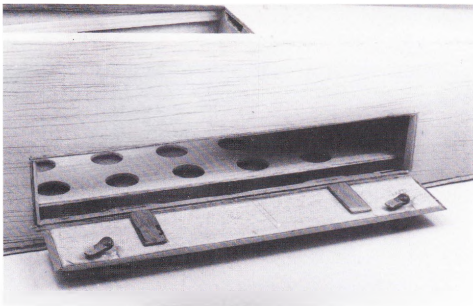
Et simpelt, men effektivt lukke til batterirummet er denne brændeskurs-mekanisme!
