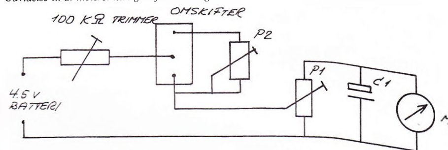
Diagram 3: Udvidelse til at meteret kan give fuldt udslag.
