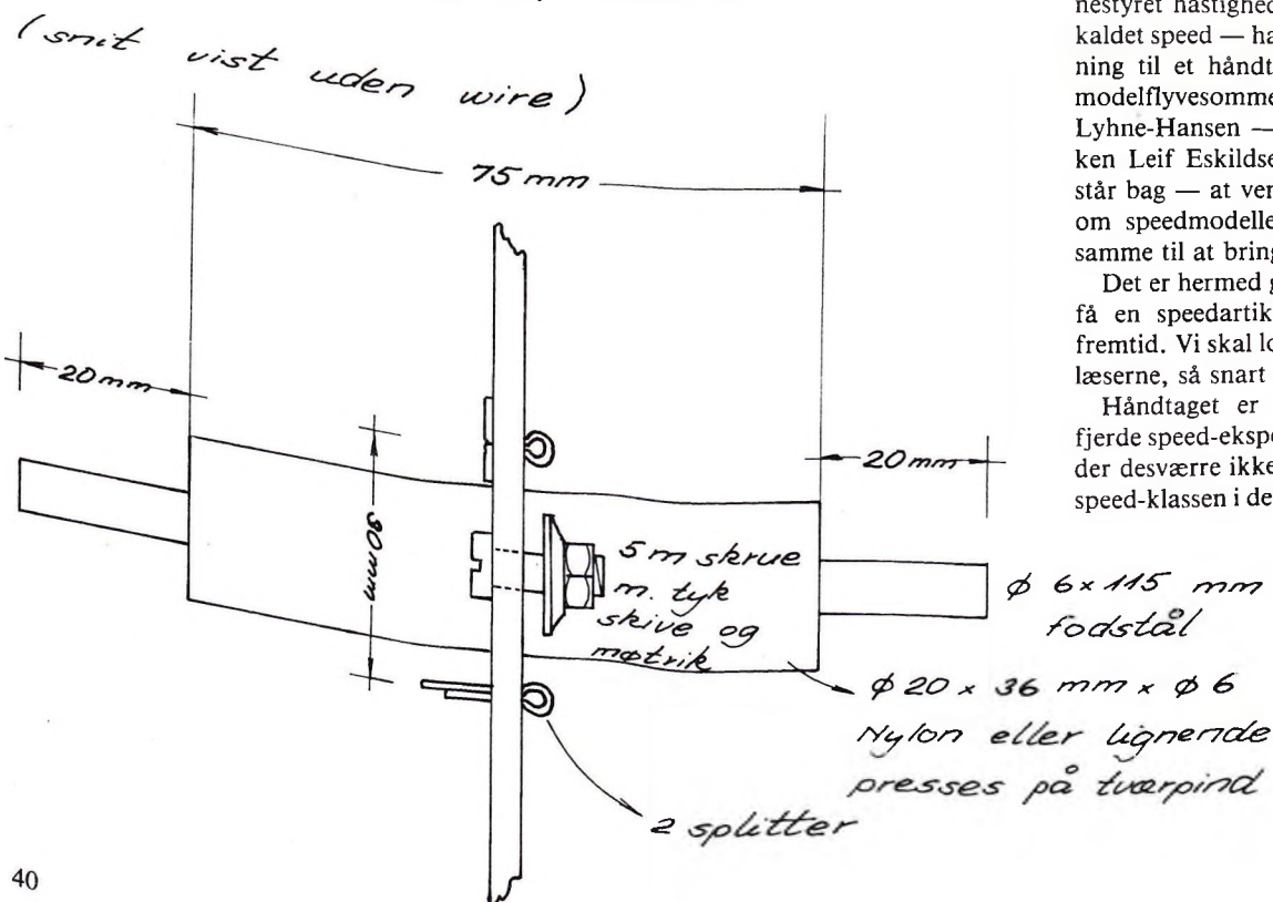
Jim Prydsø's tegning til »Bjørn Hansens patenterede referencemanipulator«, som håndtaget kaldes blandt de indviede, er i skala 1:1.
