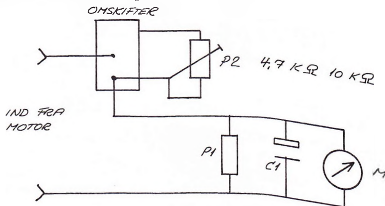
Diagram 3: Udvidelse til at meteret kan give fuldt udslag.
