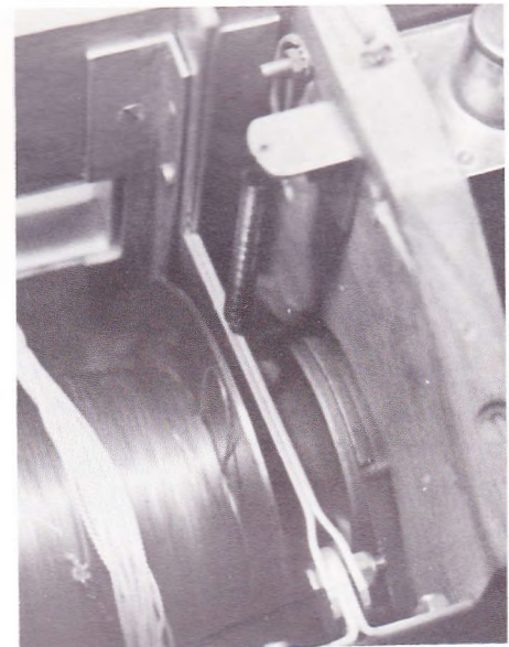
Detalje af bremsesystem, som sidder mellem motor og spiltromle. Startrelæet øverst i.h.
