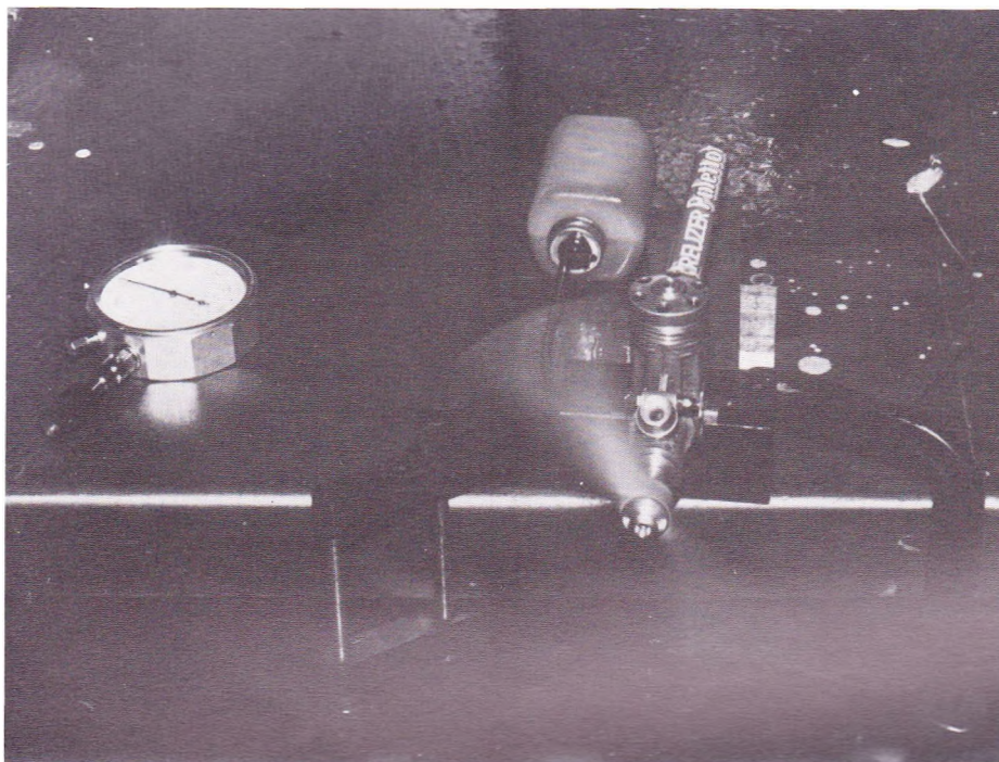
En Rossi 2,5 cm 3 ved 19.900 omdrejninger under prøvetørsel indendørs med udsugningsanlæg. Omdrejningstælleren til venstre er Henriks Hasler — et fint stykke værktøj.
