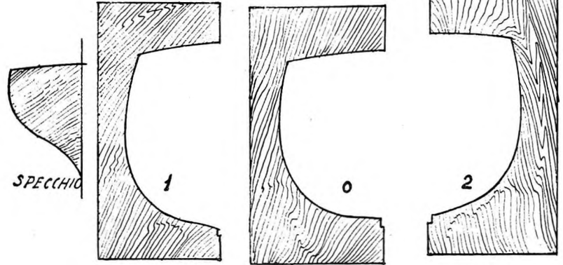
SAGOME DELLO SCAFO
