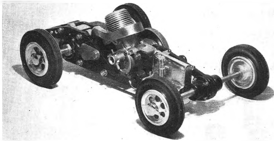
In questa foto potete ammirare il telaio dell'automodello di G. Clerici, vincitore del Gran Premio Milano, classe « C ». Il motore montato su questo modello non è però il « Mc Coy 60 », quello della vittoria, bensì il G. 17, autoaccensione da 10 cc.
