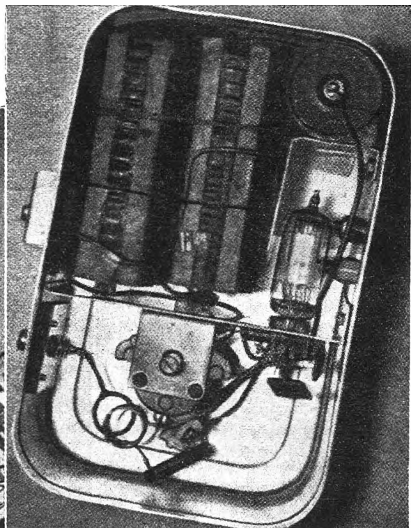
Trasmittente e ricevente sono opera dell'appassionato belga De Wals; il peso della ricevente è di soli 35 grammi, impiegando la celebre valvola R.K. 61.
