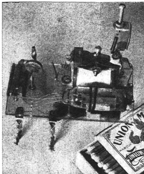
Trasmittente e ricevente sono opera dell'appassionato belga De Wals; il peso della ricevente è di soli 35 grammi, impiegando la celebre valvola R.K. 61.
