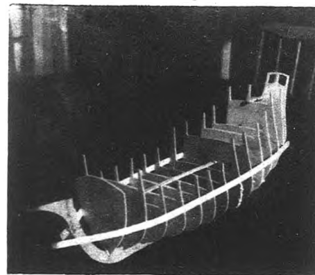
Ecco come si presenta lo scheletro del nostro modello dopo che avrete seguito a puntino tutte le nostre istruzioni
