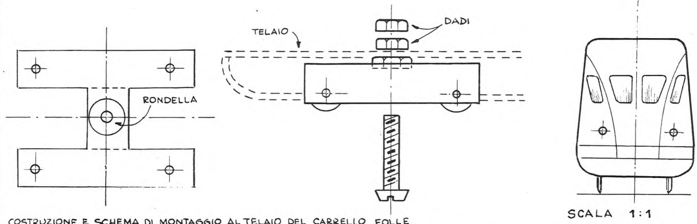
COSTRUZIONE E SCHEMA DI MONTAGGIO AL TELAIO DEL CARRELLO FOLLE
