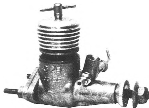
G. 29 - Cilindrata 0,8 cc. Corsa mm. 8,5. Alesaggio mm. 11,1. Peso gr. 43. Tipo diesel e tipo glow-plug. Regime di rotazione 14.000 giri con elica 15,5x7,5.
