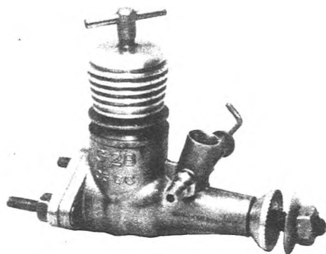
G. 28 - Cilindrata 0,5 cc. Corsa mm. 8,5. Alesaggio mm. 8,5. Peso gr. 38. Tipo diesel e tipo glow-plug. Regime di rotazione 15.000 giri con elica da 13x7,5.
